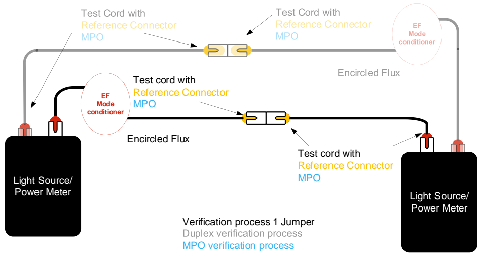
«one Jumper» method verification
