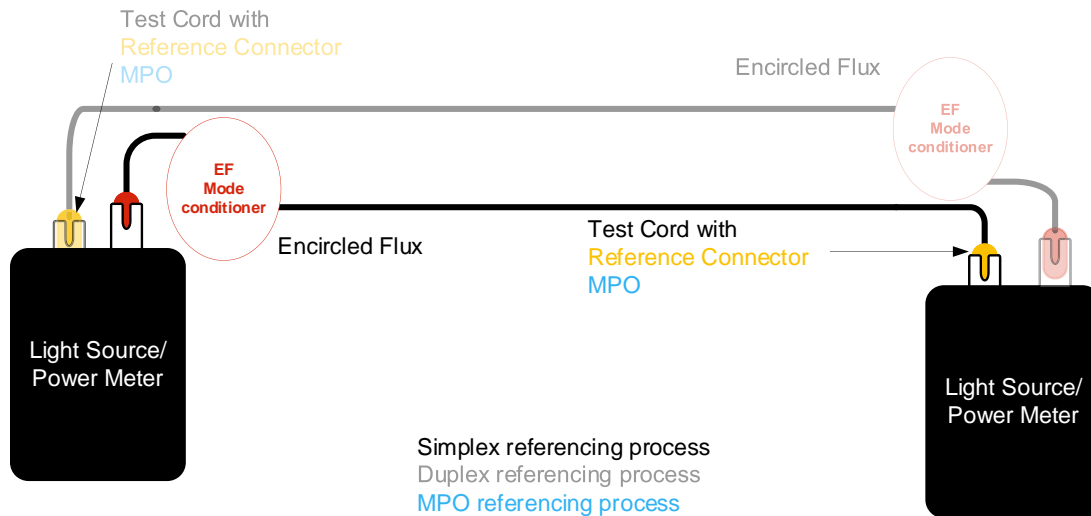
«one Jumper» reference method
